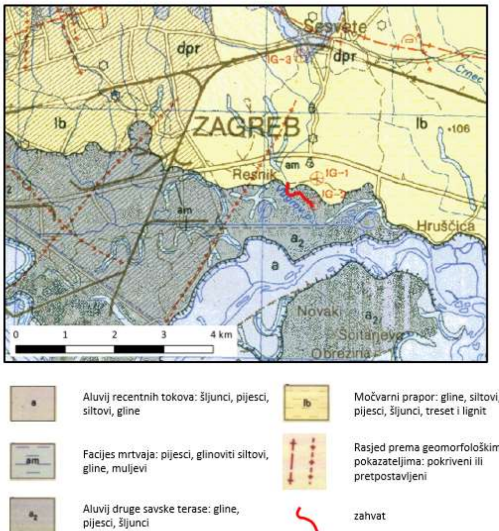
Slika 3.1.3-1. Geološka karta šireg područja zahvata s ucrtanim zahvatom (izvor: Basch i dr., 1981. )
